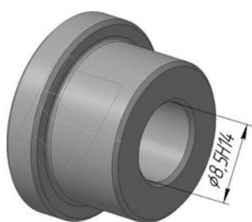
Рис. 19. Втулка Ø8,5H14 и выборка по внутреннему диаметру втулки - в ячейке A1 введем текст «Номер изделия», и пронумеруем от 1 до 100.
