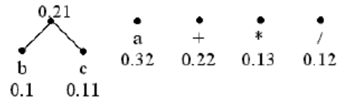
2) Слияние поддеревьев с весами 0.1 и 0.11
