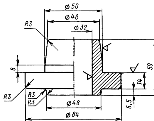
вариант 9 Букса
