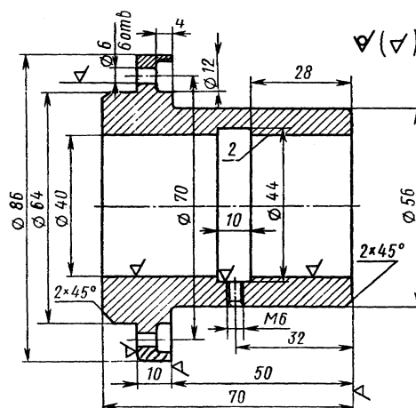
вариант 7 Корпус
