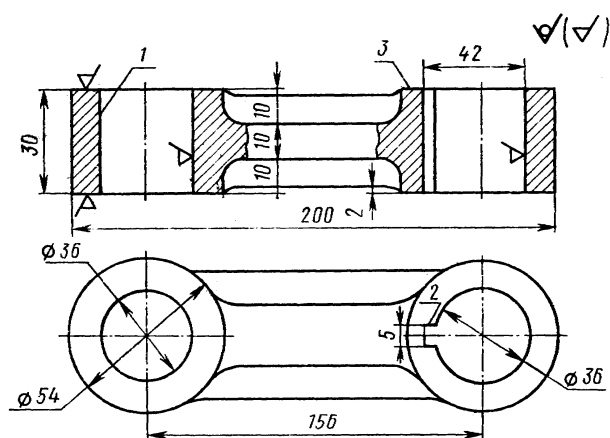
вариант 1 Траверса
