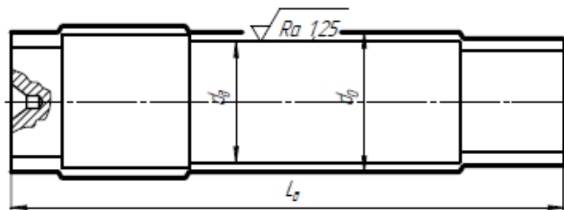
Рис. 2.4. Эскиз заготовки
