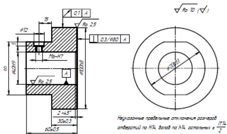
Рис. 2.6. Операционный эскиз
