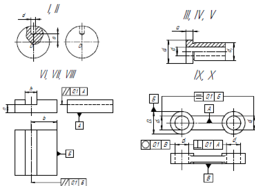
Рис. 1.5. Операционные эскизы
