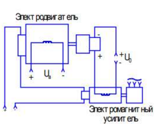
Рис. 9. Принципиальная схема регулирования числа оборотов двигателя (вариант 5)
