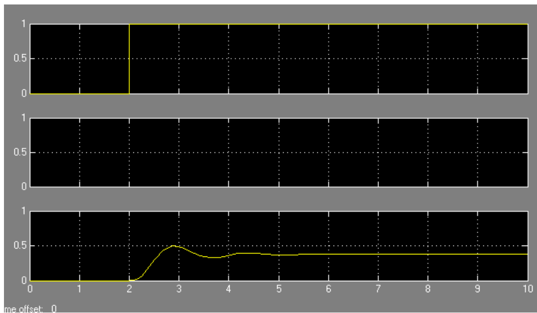
Рис.10. Переходной процесс системы по задающему воздействию
