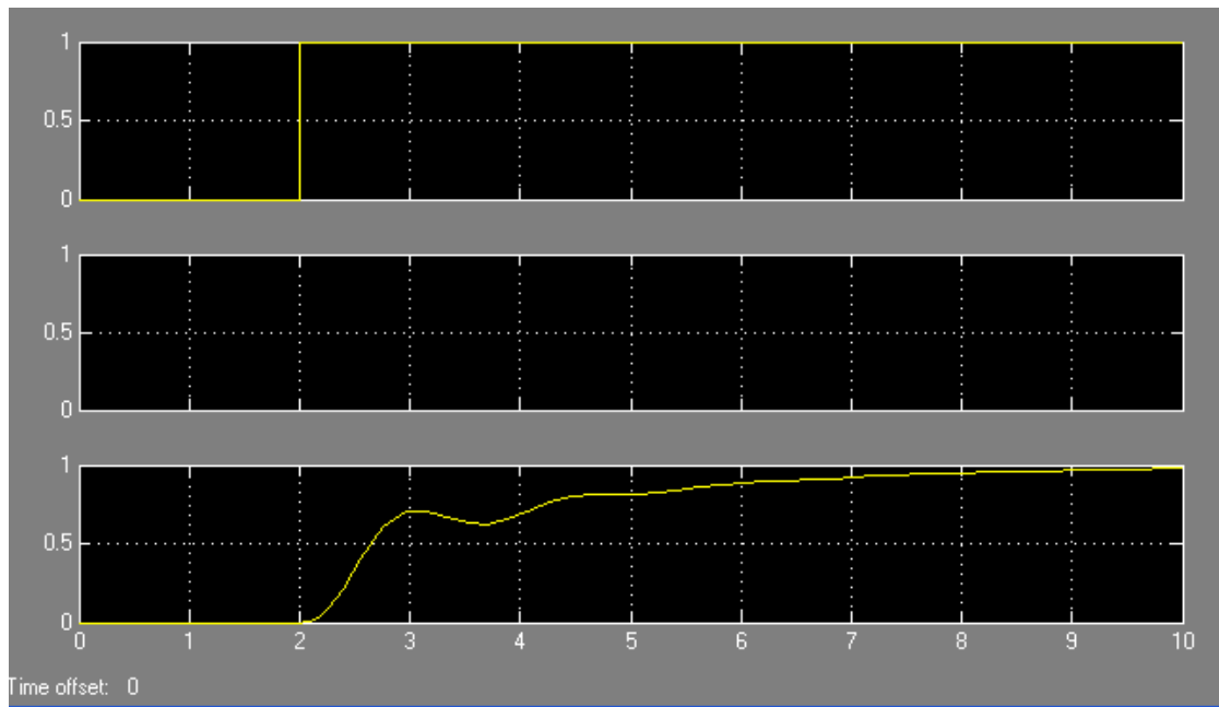
Рис.11. Переходной процесс системы по задающему воздействию
