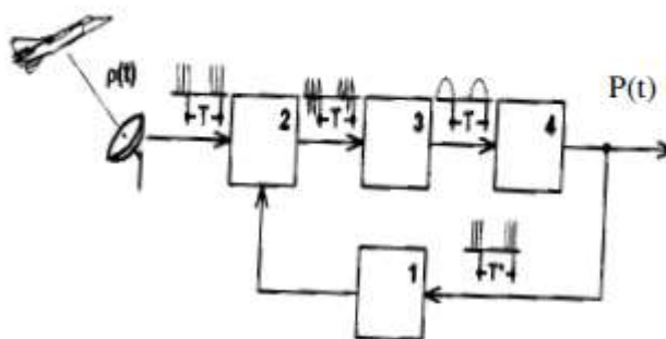
Рис. 28. Система определения расстояния от радиолокационной станции до подвижной цели (вариант 24)
