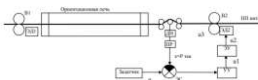
Рис. П14. Функциональная схема системы управления силой натяжения волокна при ориентационной вытяжке путем корректировки скорости вальцев на выходе
