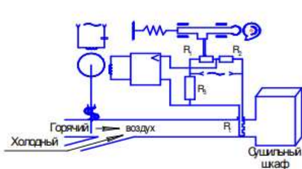
Рис.17. Принципиальная схема регулирования температуры в сушильном шкафе (вариант 13)
