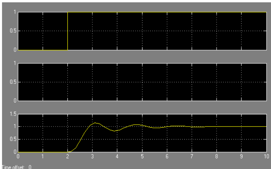
Рис.12. Переходной процесс системы по задающему воздействию
