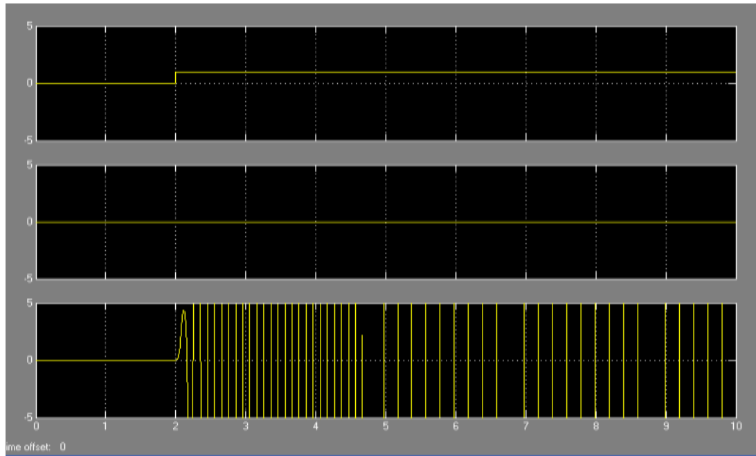
Рис.9. Переходной процесс системы по задающему воздействию при k_p = 1, k_i = 0, k_d = 0
