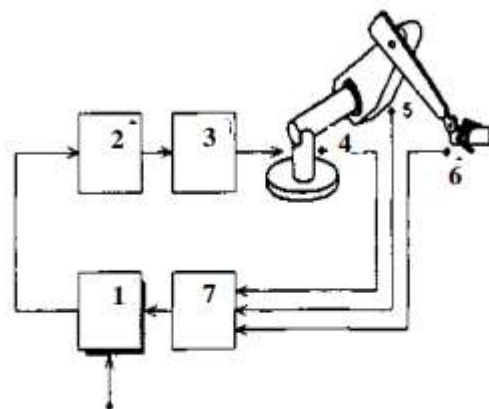
Рис. 26. Система управления движением манипуляционным роботом (вариант 22)
