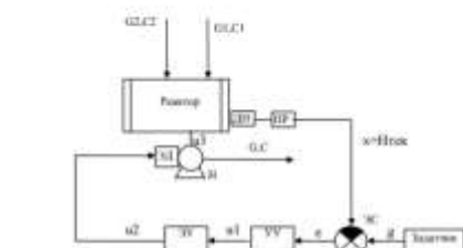
Рис. П13. Функциональная схема системы управления уровнем реагента путем корректировки расхода на входе
