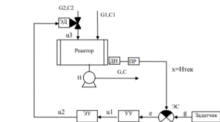
Рис. П11. Функциональная схема системы управления уровнем реагента путем корректировки расхода на входе
