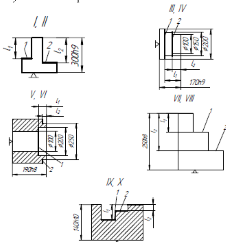
Рис. 1.7. Варианты для расчета размерных цепей
