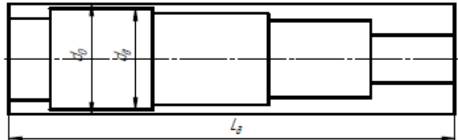
Рис. 2.3. Заготовка – круг
