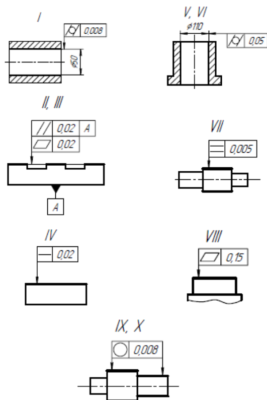
Рис. 1.3 Операционные эскизы
