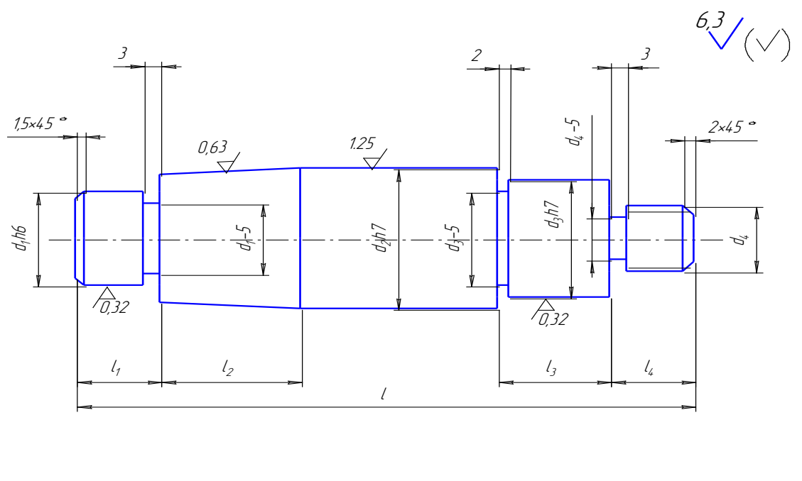
Рис. 1. Типовая деталь.
