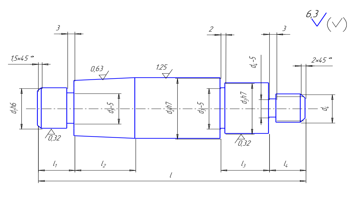
Рис. 1. Типовая деталь.
