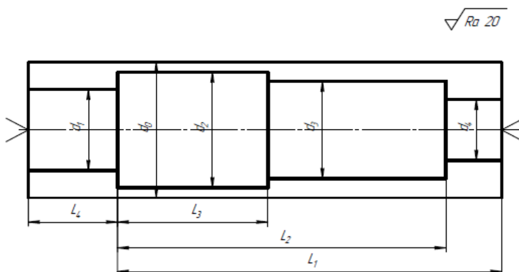
Рис. 2.7. Эскиз детали
