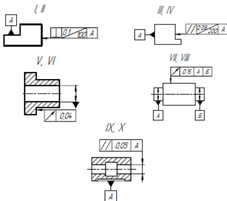
Рис. 1.4. Варианты обработки поверхностей
