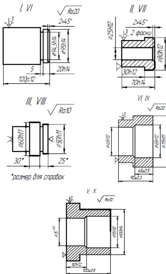
Рис. 1.1 Операционные эскизы
