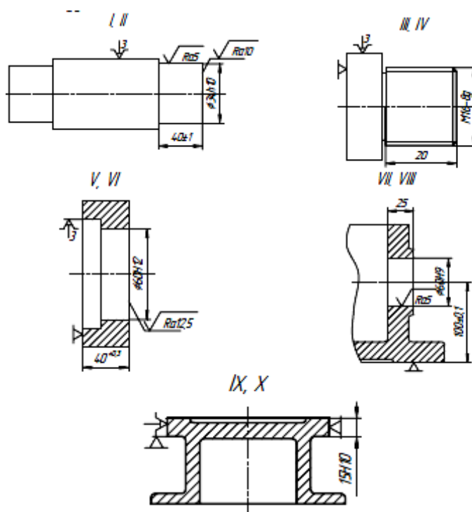
Рис. 1.2 Операционные эскизы
