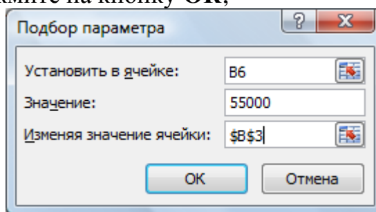
Рисунок 8 – Ввод параметров
